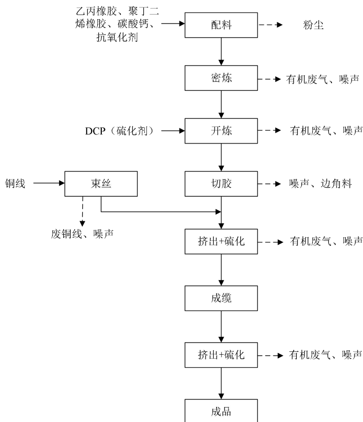
图 2-4. 橡胶电缆生产工艺流程图
