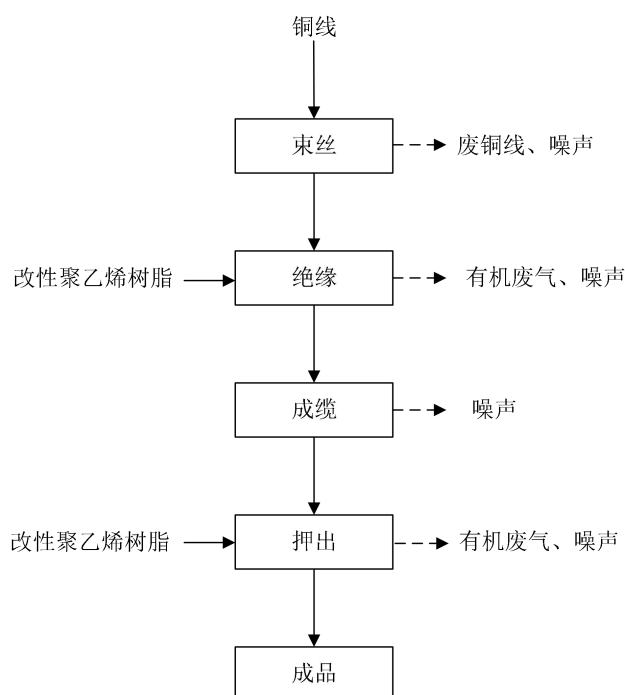
图 2-3. 塑料电缆生产工艺流程图
