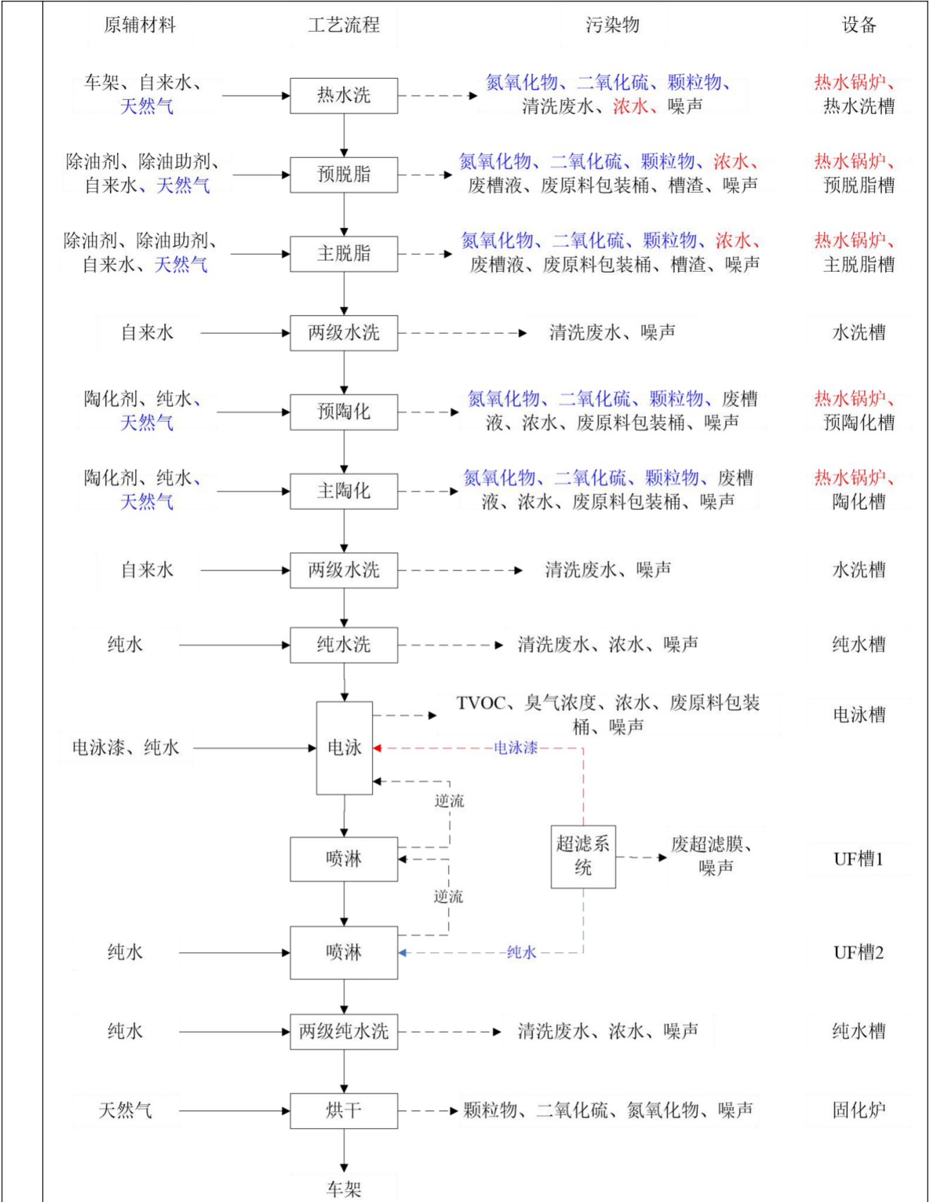
图 2-7 车架加工生产工艺流程及产污环节图
