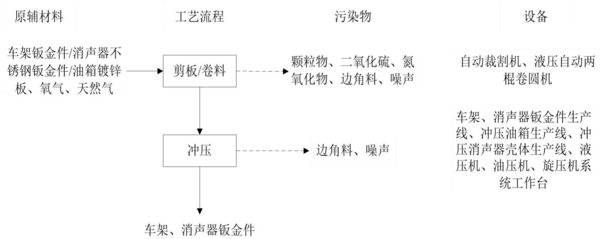
图 2-4 车架、消声器钣金件生产线工艺流程及产污环节图 工艺流程说明：
