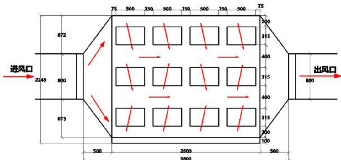
图 4-2a 本项目单级活性炭箱结构侧视图
