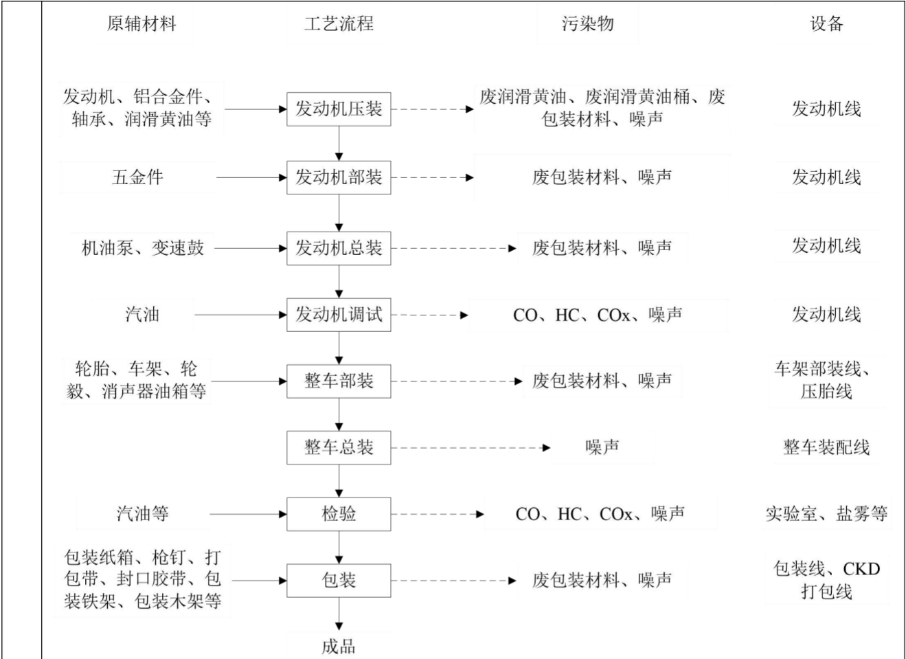
图 2-8 总装工艺流程及产污环节图
