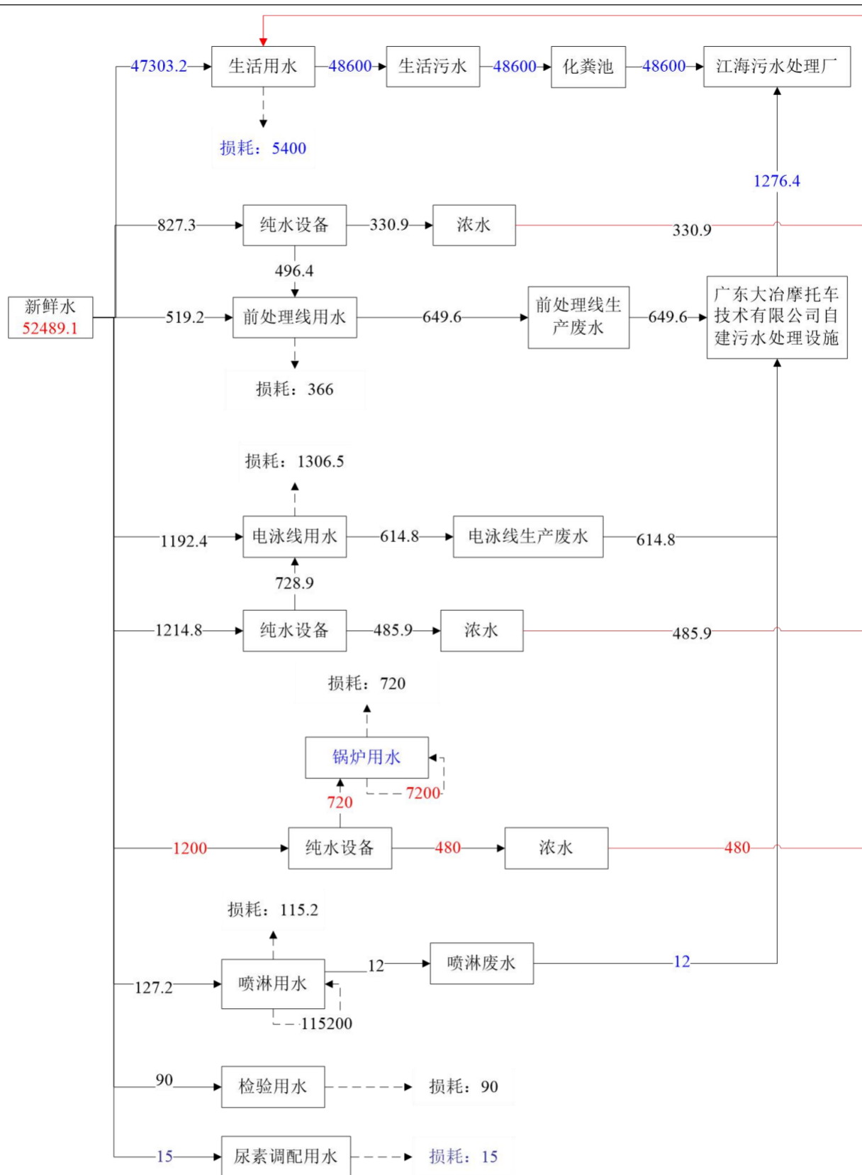
图 2-1 项目水平衡图 单位: m³/a
