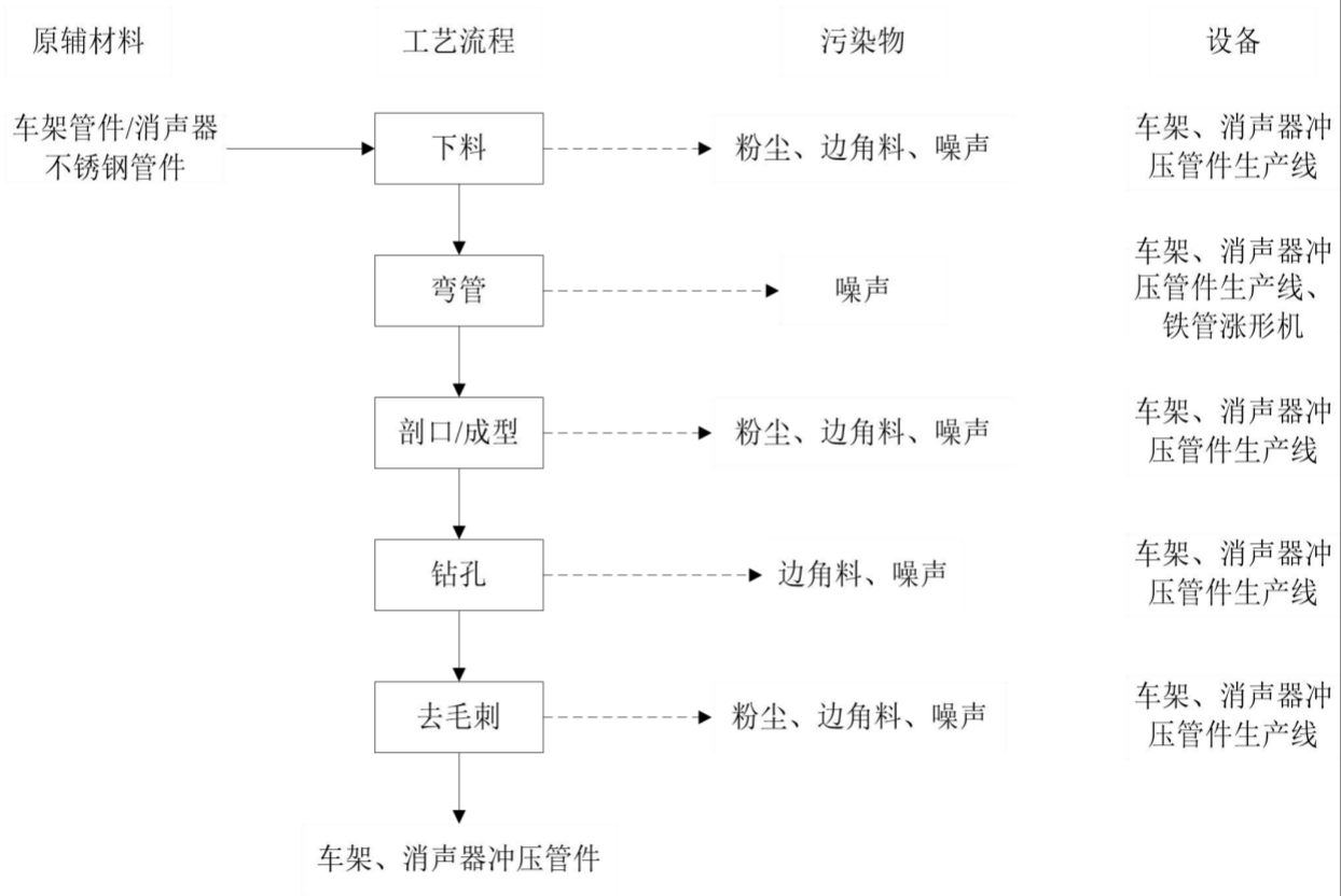
图 2-3 车架、消声器管件生产线工艺流程及产污环节图 工艺流程说明：
