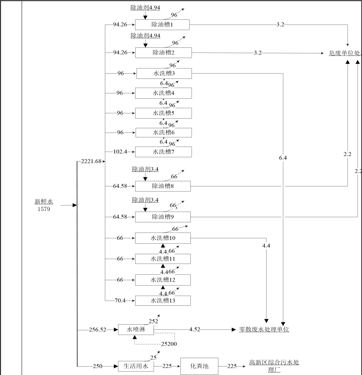
图 2-2 项目年水平衡图 (单位: 吨/年)
