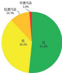
图1 2024年度国家网空气质量类别分布
