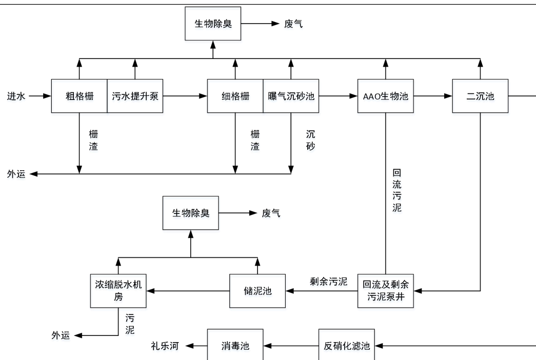
图 4-1 江门高新区综合污水处理厂废水处理工艺流程图
