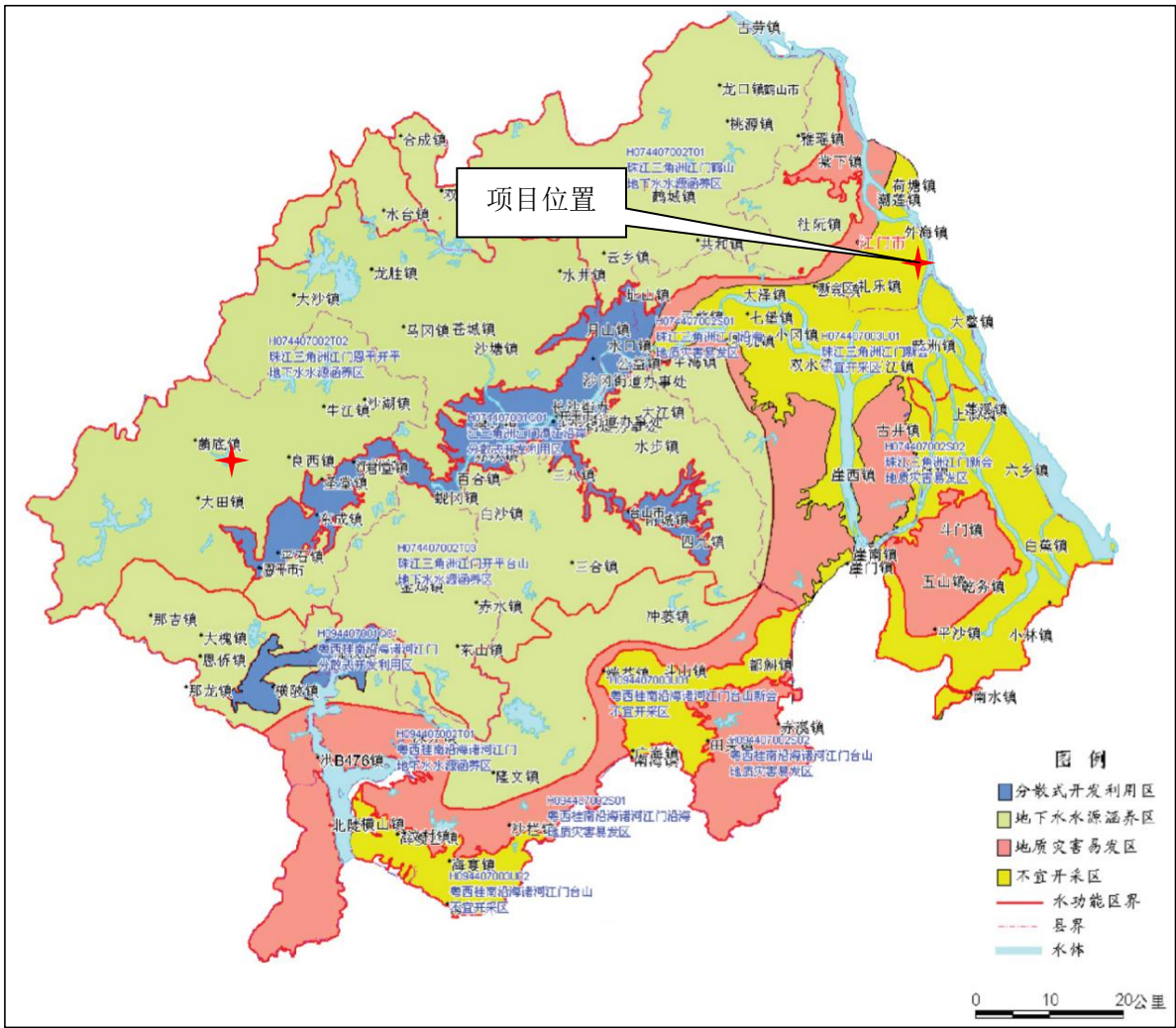
附图 5 项目所在区域地下水环境功能区划图
