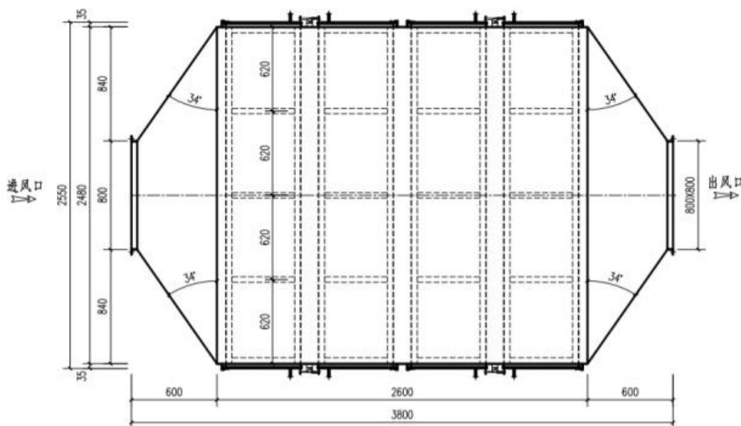
图 4-2 本项目单级活性炭箱结构俯视图
