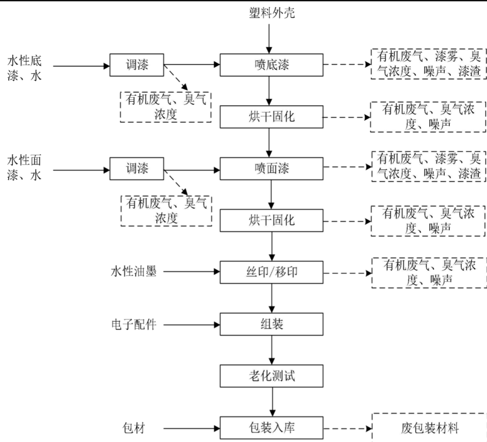
图 2-6 台钟工艺流程图及产污节点图
