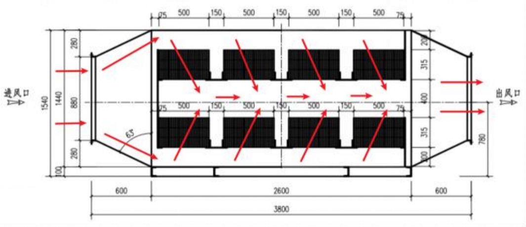
图 4-1 本项目单级活性炭箱结构侧视图
