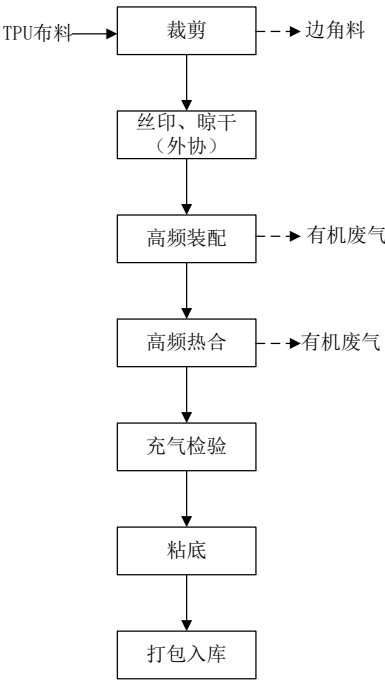
图2-2. 项目工艺流程图
