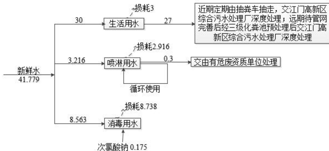
(4) 水平衡图（单位：t/a）
