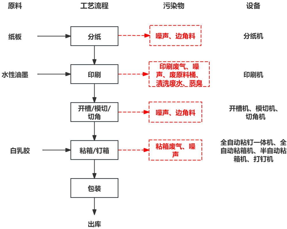
图 2-2 纸箱工艺流程图及产污节点图
