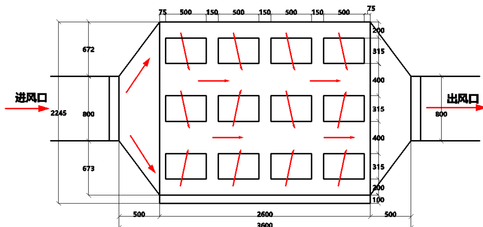
图 4-1 本项目单级活性炭箱结构侧视图
