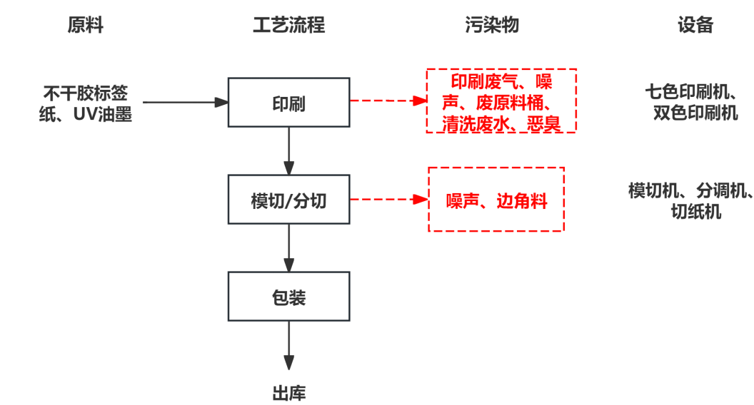
图 2-3 不干胶标贴工艺流程图及产污节点图
