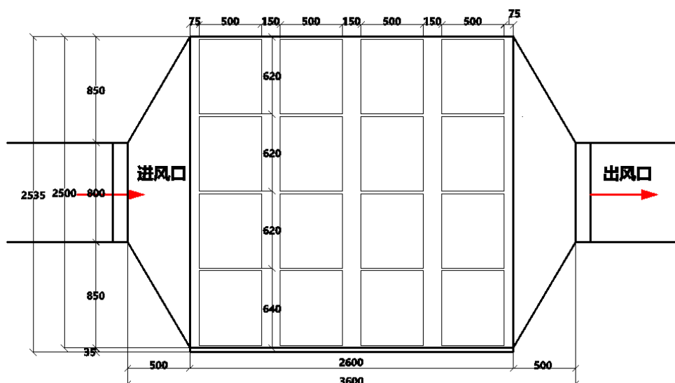
图 4-2 本项目单级活性炭箱结构俯视图
