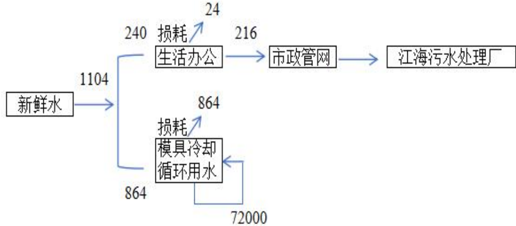
图 2-1 水量平衡图(t/a)
