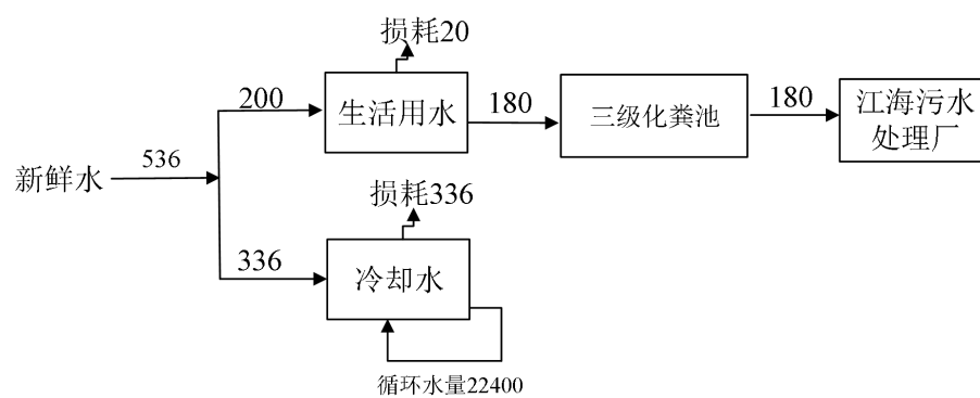
图 2-1 项目水平衡图 (m³/a)
