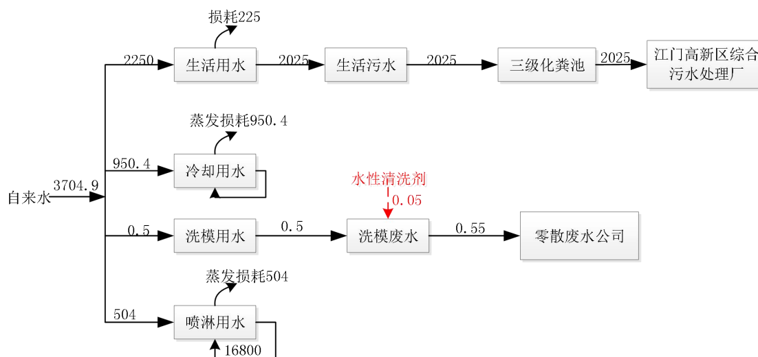
图 1 水平衡图
