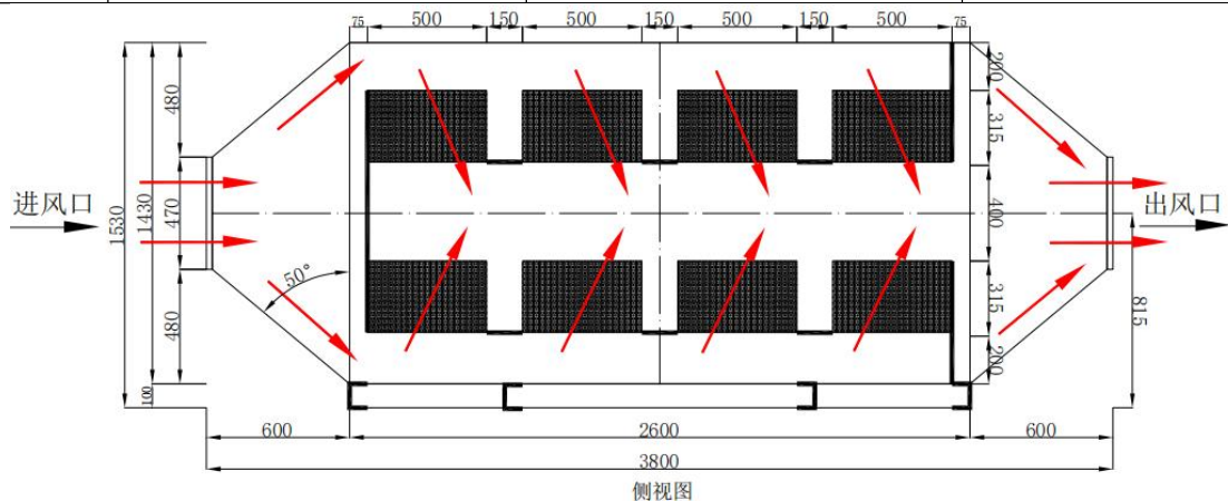
图 4-3b 本项目单级活性炭箱结构侧视图
