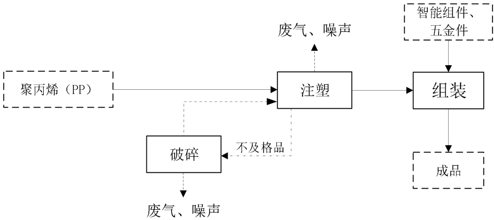
图 2-2 智能筒灯生产工艺流程及产污环节图
