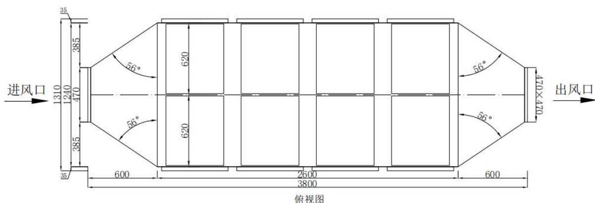
图 4-3b 本项目单级活性炭箱结构俯视图
