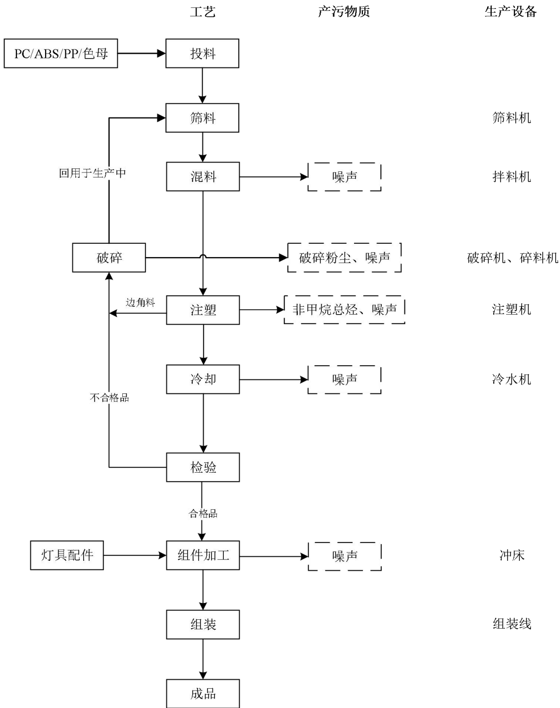
图 2-2 蜂窝灯生产工艺流程及产污环节图
