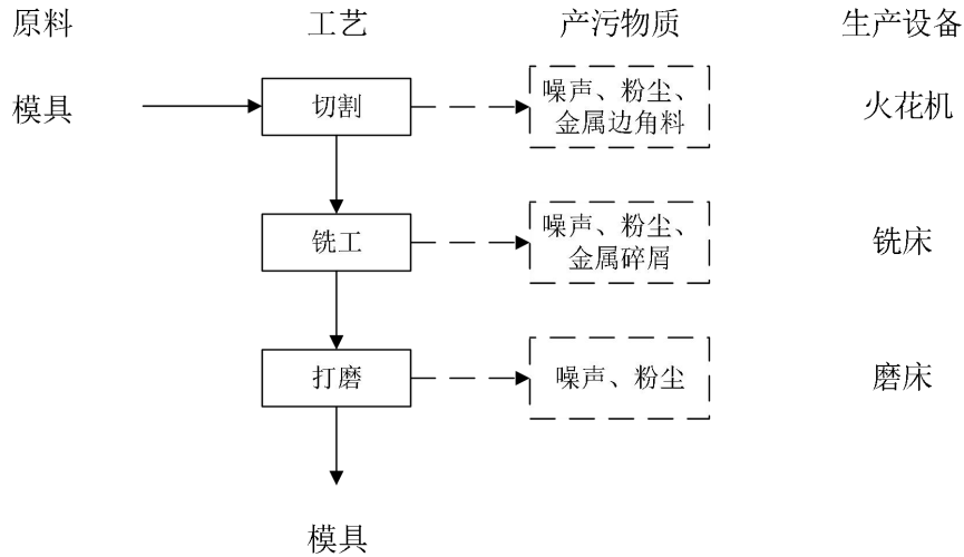
图 2-3 模具修理工艺流程及产污环节图
