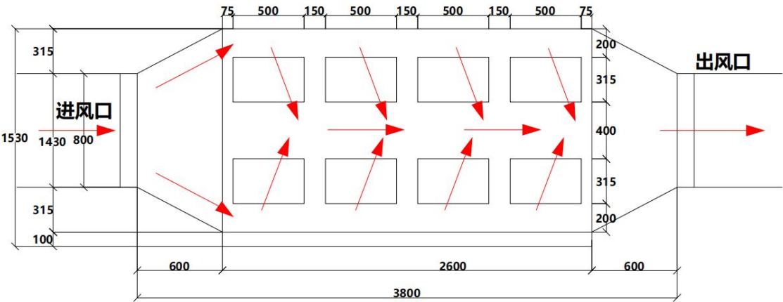
图 4-2 单级活性炭吸附装置结构侧视图
