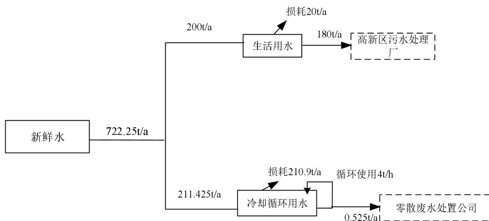
图 2-2 扩建项目水平衡图
