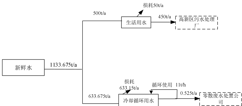
图 2-4 扩建后全厂水平衡图
