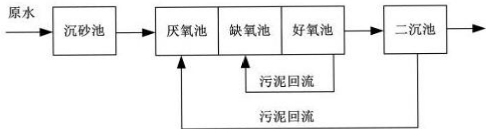
图 4-1 江门高新区综合污水处理厂污水处理工艺
