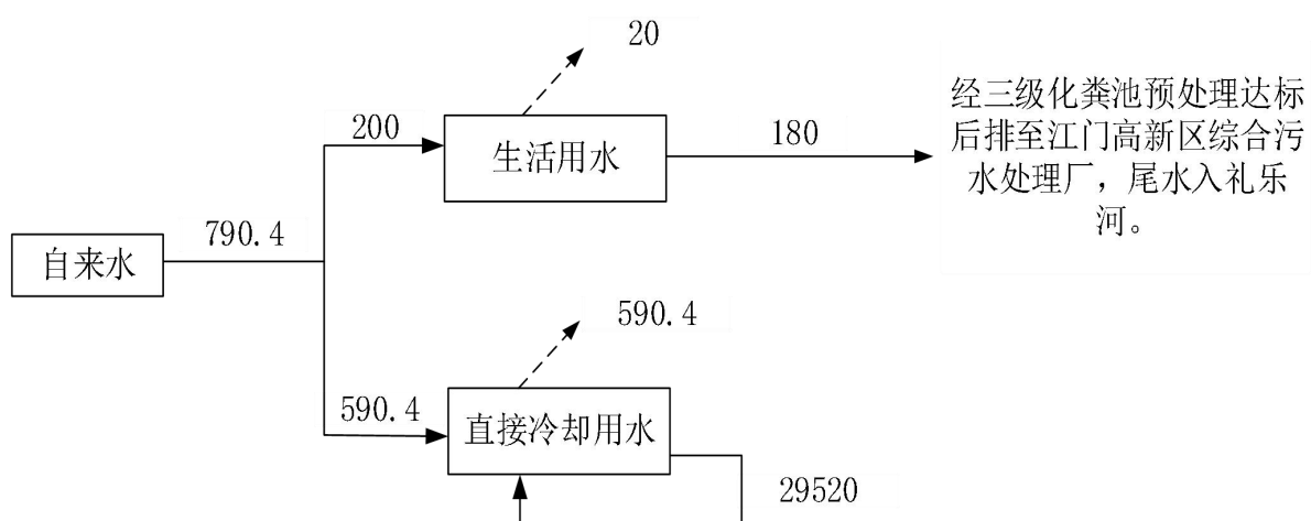
图 2-1 全厂用水平衡图（单位：t/a）
