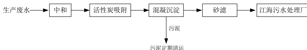
图 3. 废水处理工艺流程图
