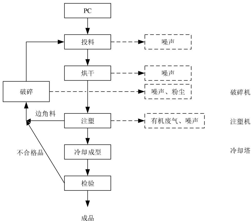
图 2. 生产工艺流程图
