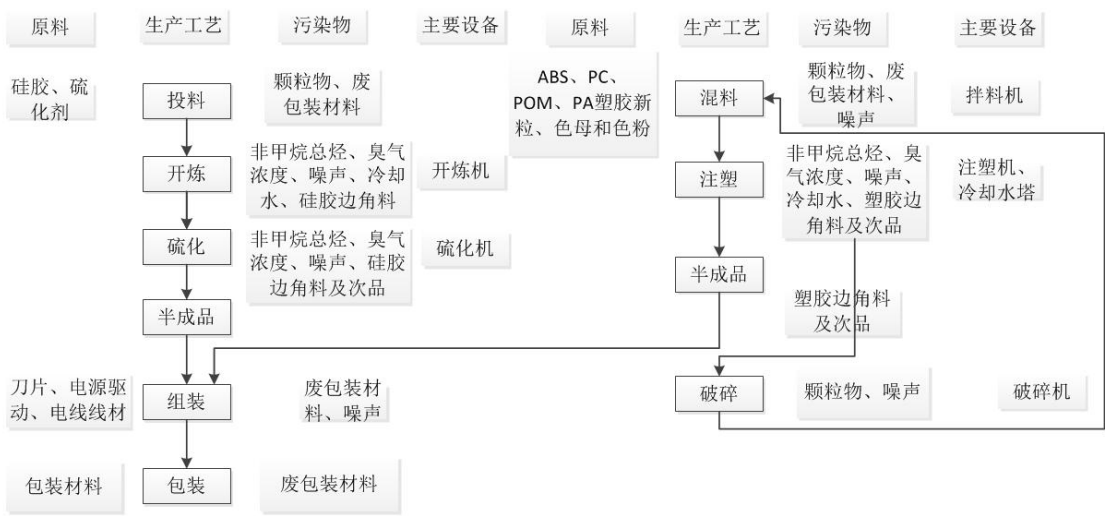
图 2-1 果汁榨汁机生产工艺流程图
