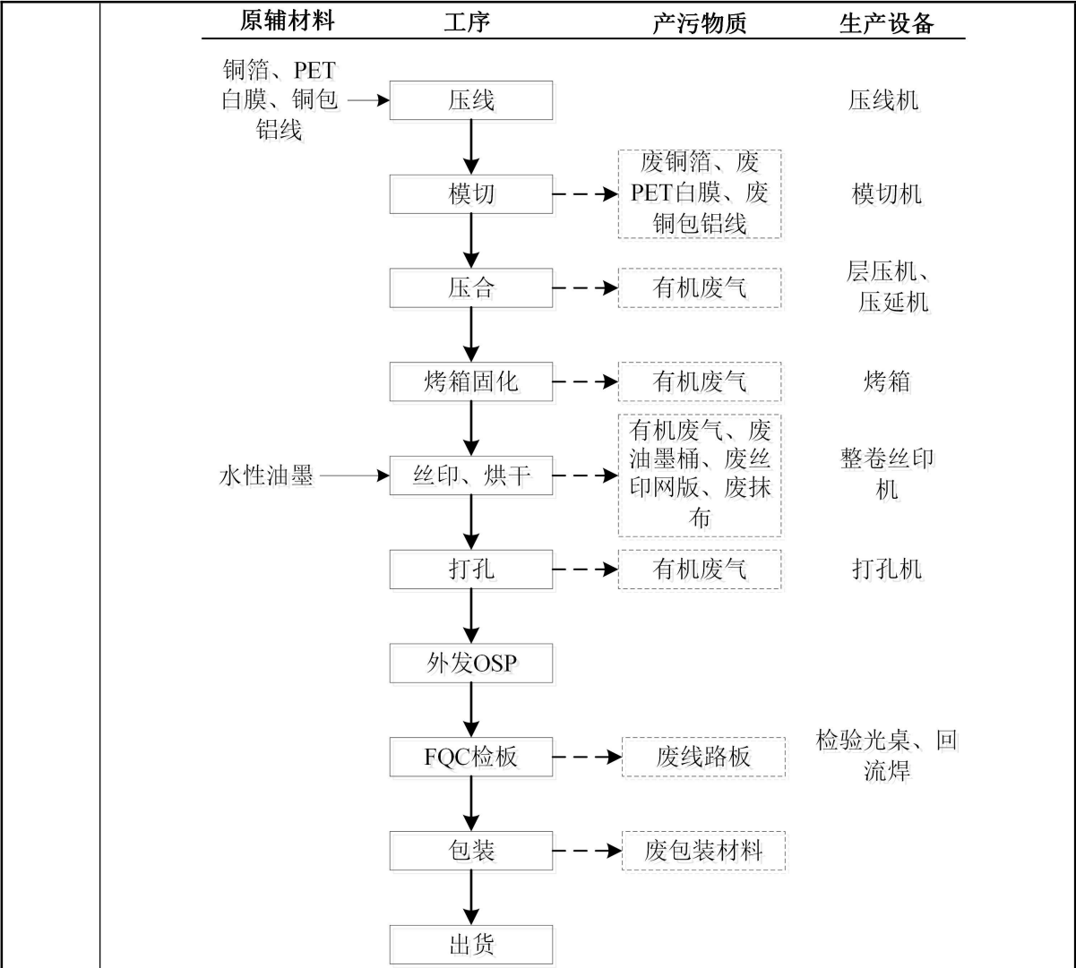
图 2-2 项目生产工艺流程图
