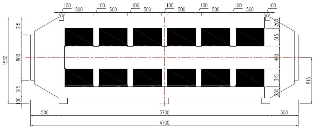
图 4-1 活性炭吸附箱正视图
