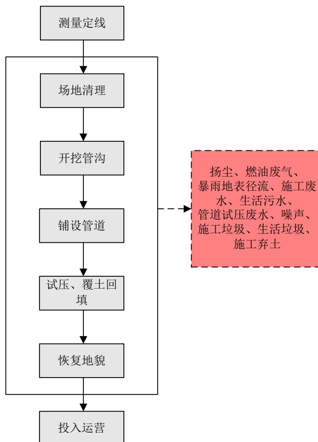
图 2-3 本项目管道施工工艺流程图
