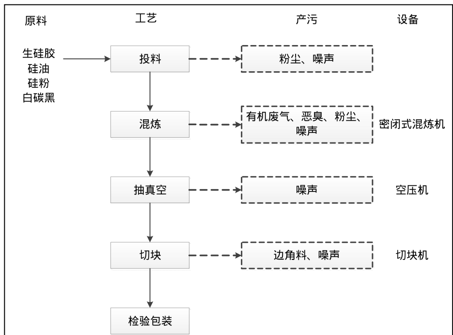
图 2-2 硅胶混炼胶生产工艺流程图
