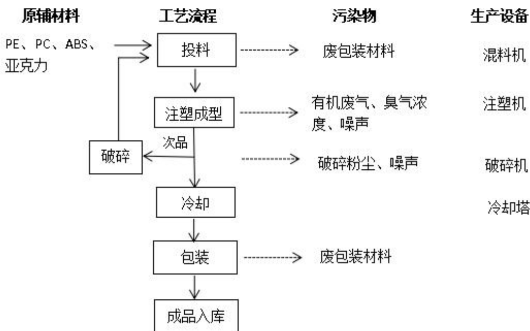
图 2-2 项目灯饰塑料配件生产工艺流程图
