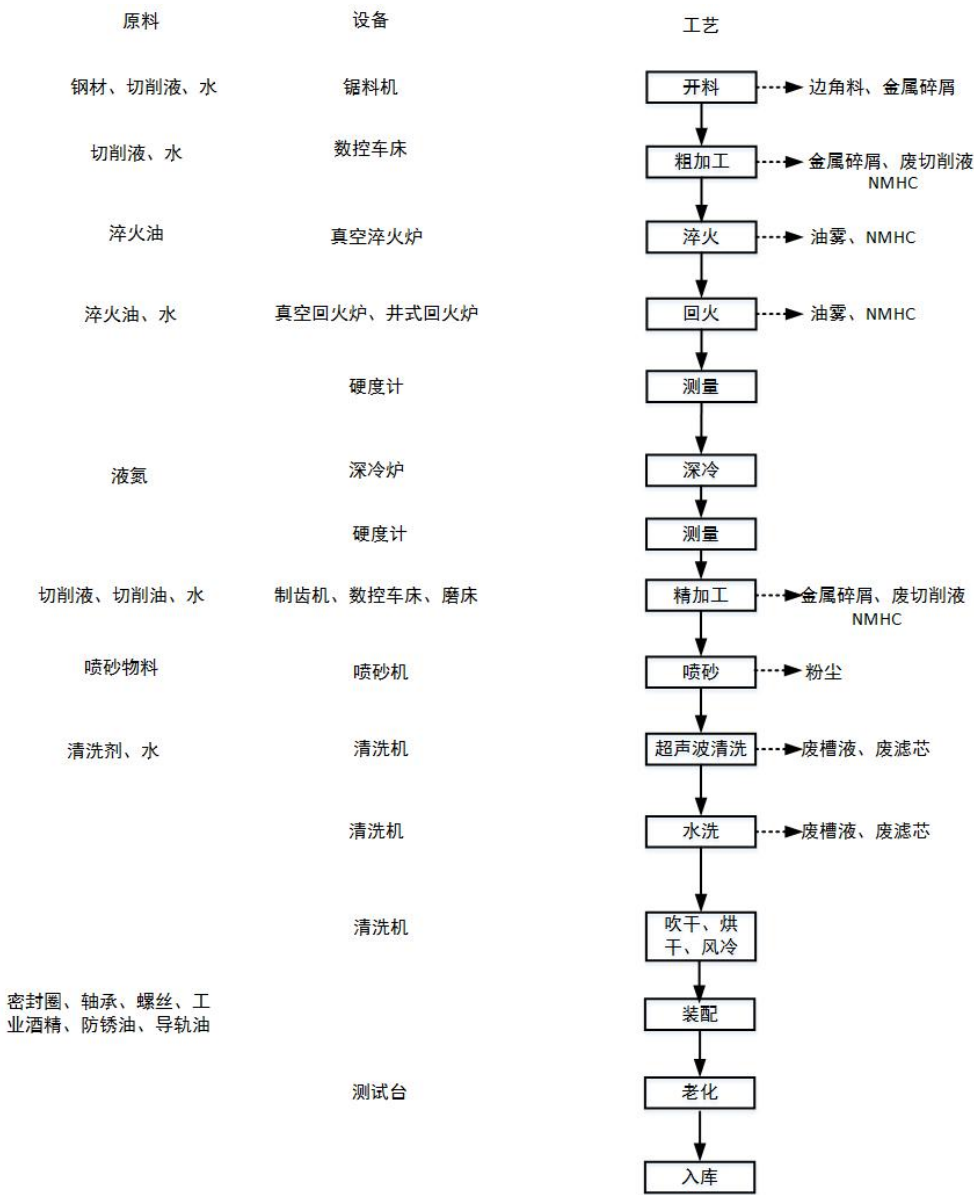
图 2-5 改扩建前项目工艺流程图
