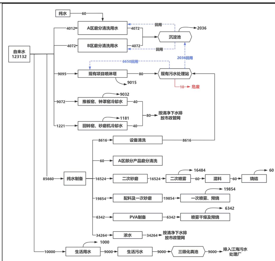
图 2-4 现有项目水平衡图
