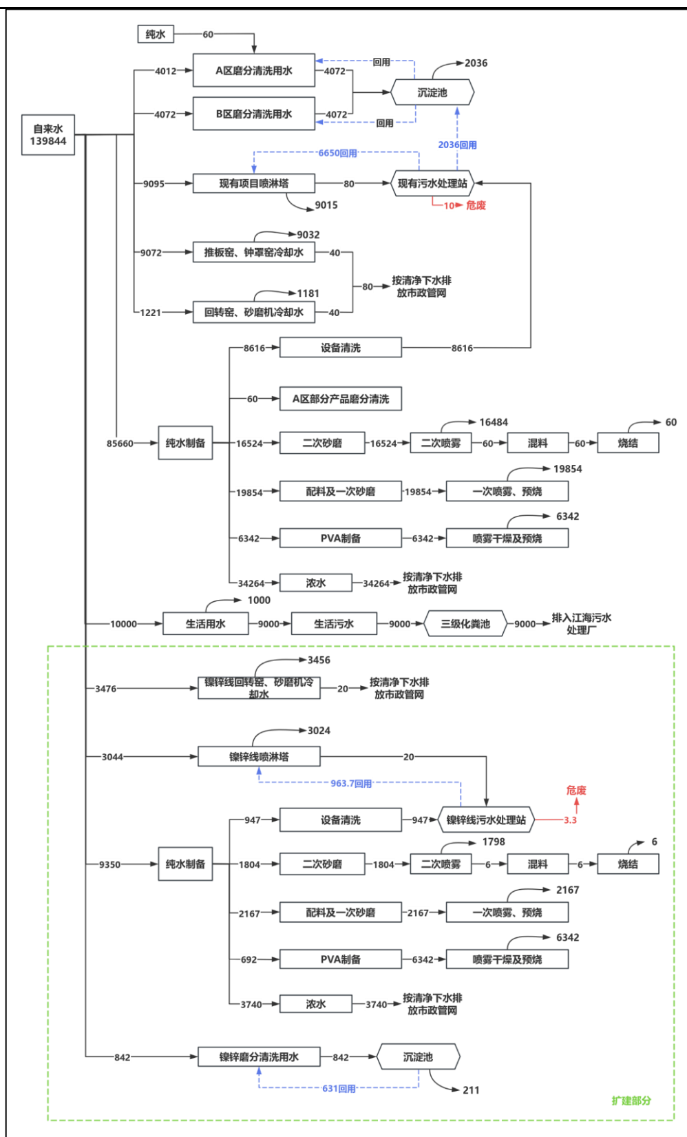
图 2-1 本项目改扩建后全厂水平衡图
