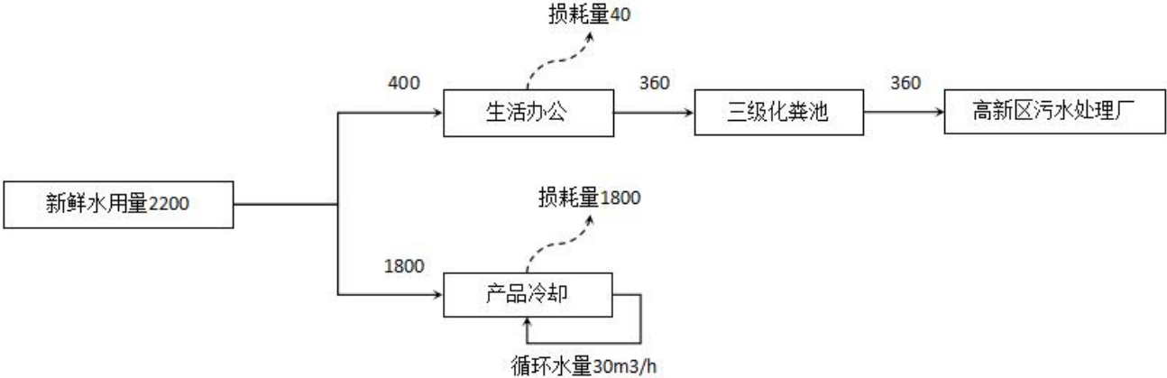
图 2-1 项目水平衡图 (t/a)
