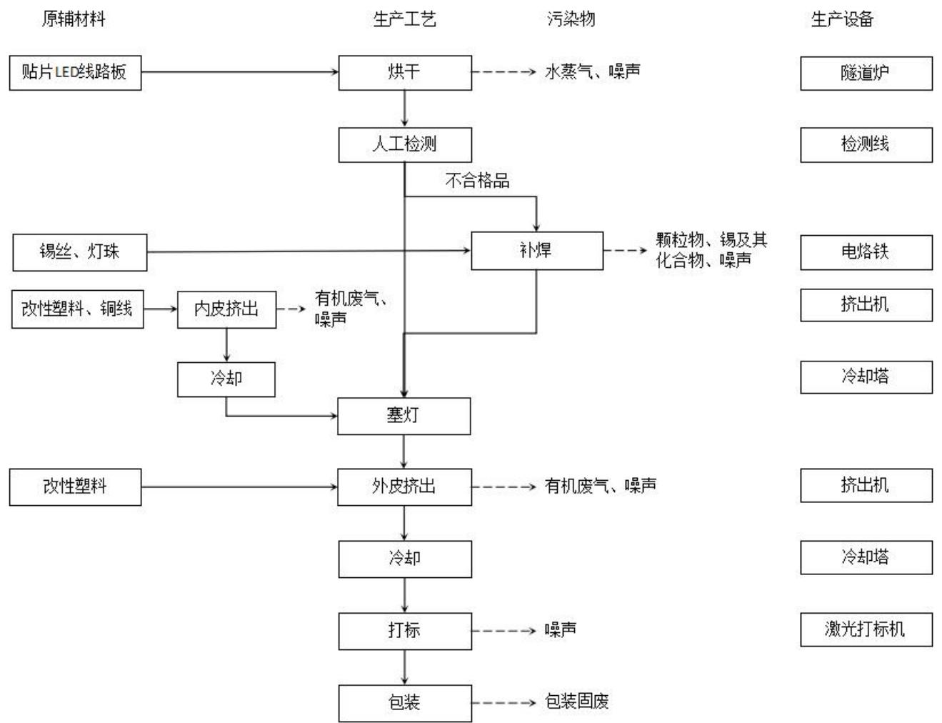
图2-3 LED灯带生产工艺流程图
