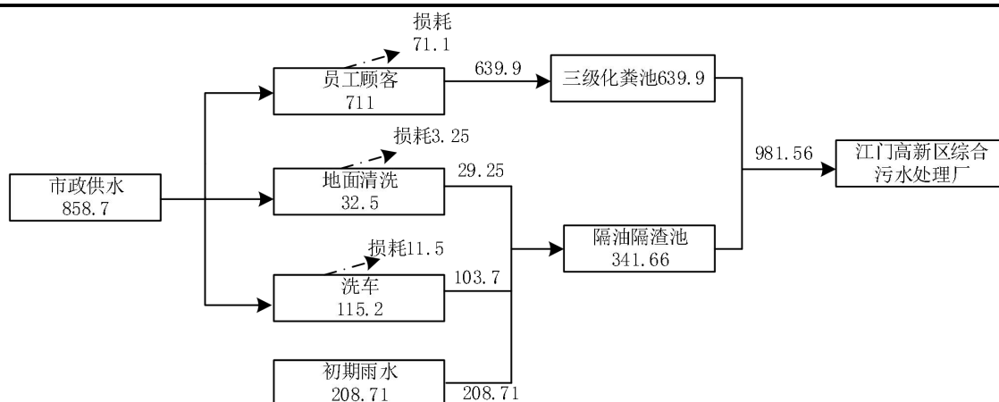
图 2-1 改扩建后项目水平衡图（单位：m³/a）
