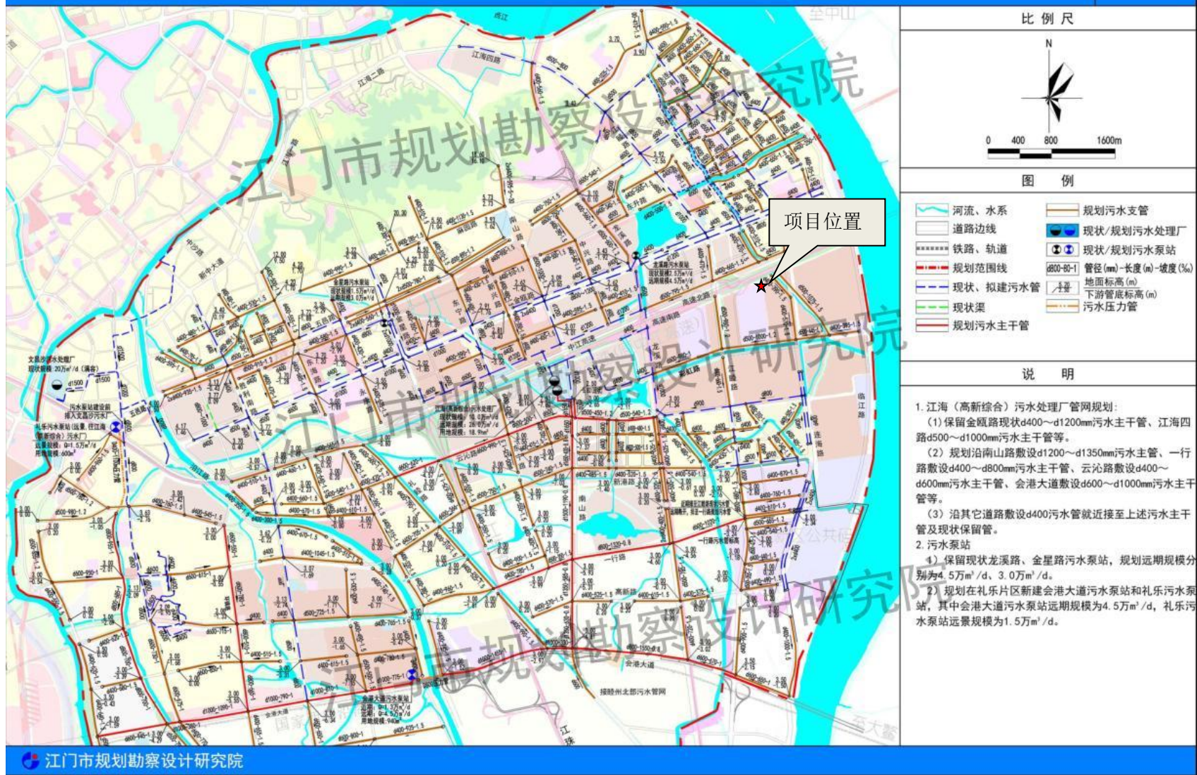
附图 13 江门高新区综合污水处理厂收集系统规划图
