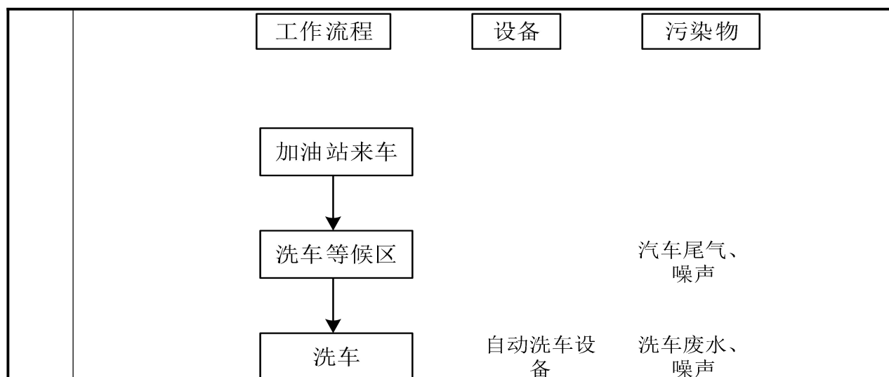
图 2-6 洗车工艺流程图
