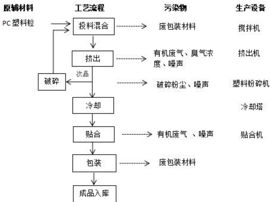
图 2-2 项目灯饰配件产工艺流程图
