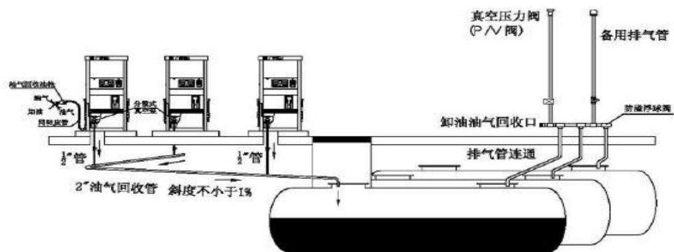
图 4-1 油罐车卸油时油气回收过程示意图
