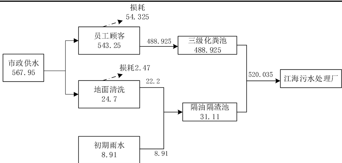
图 2-1 改扩建后项目水平衡图 (单位: t/a)
