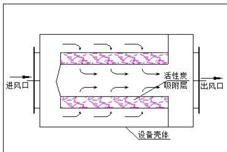
图 4-1 活性炭箱结构图
