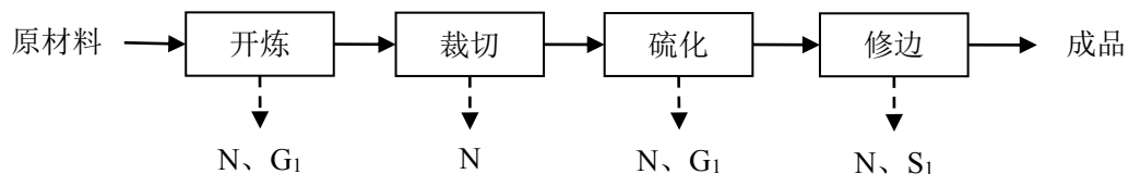
图2-2 项目生产工艺流程图
